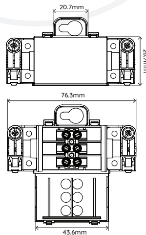
Boîtier de connexion IP44 | IP44 wire connector box
