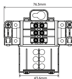
Boîtier de connexion IP44 | IP44 wire connector box
