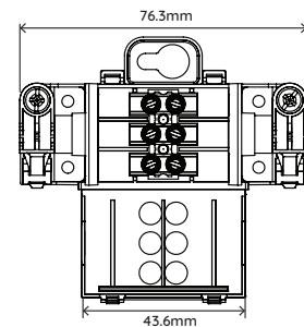
Boîtier de connexion IP44 | IP44 wire connector box
